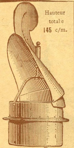
MODÈLE B Base ronde, diamètre 55 c/m
