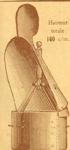
MODÈLE D Pour tuyaux. Diamètre 60 c/m
